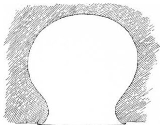
Fig. 7. Tillese. Snit af lydpotte i apsishvælvet. 1:5. (S. 342).
