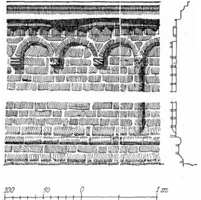
Fig. 4. Tillese. Detaljer fra Apsis. 1:50. Målt af Elna Møller 1948.
