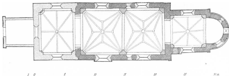
Fig. 2. Tillese. Plan. 1:300. Målt af C. G. Schultz 1948.
